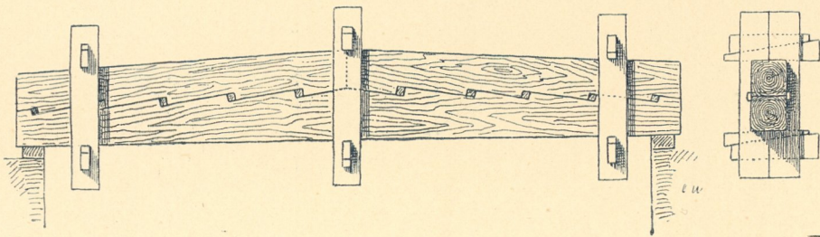
Fig. 83. Verzahn ter Träger.
