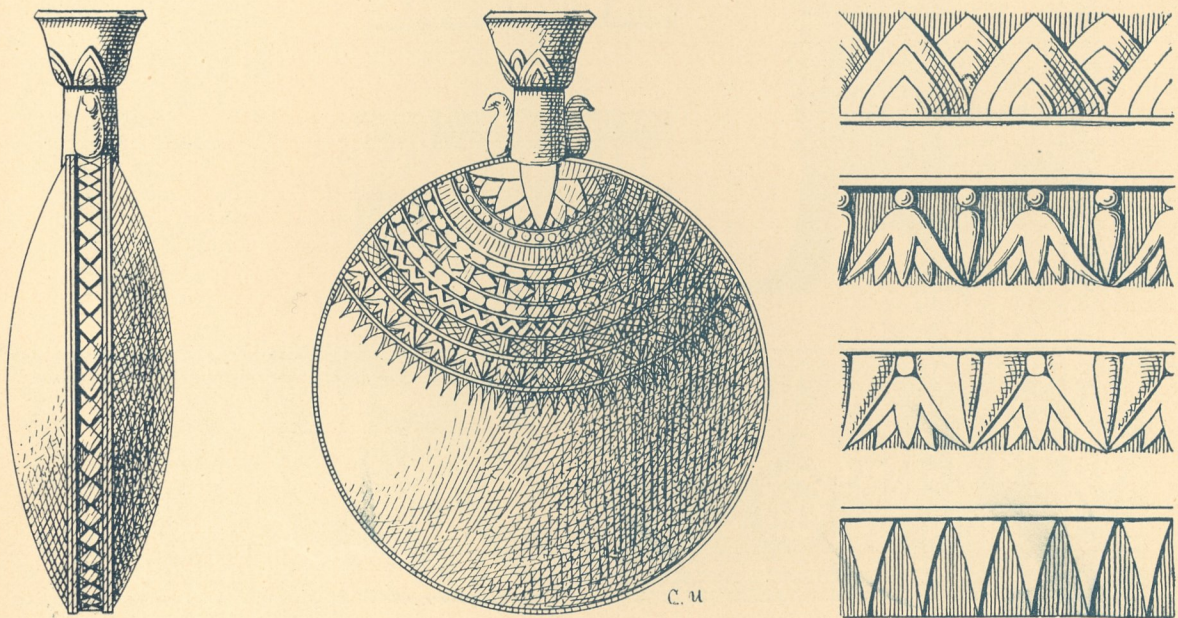
Fig. 21. Altägyptisches Glasflacon.
