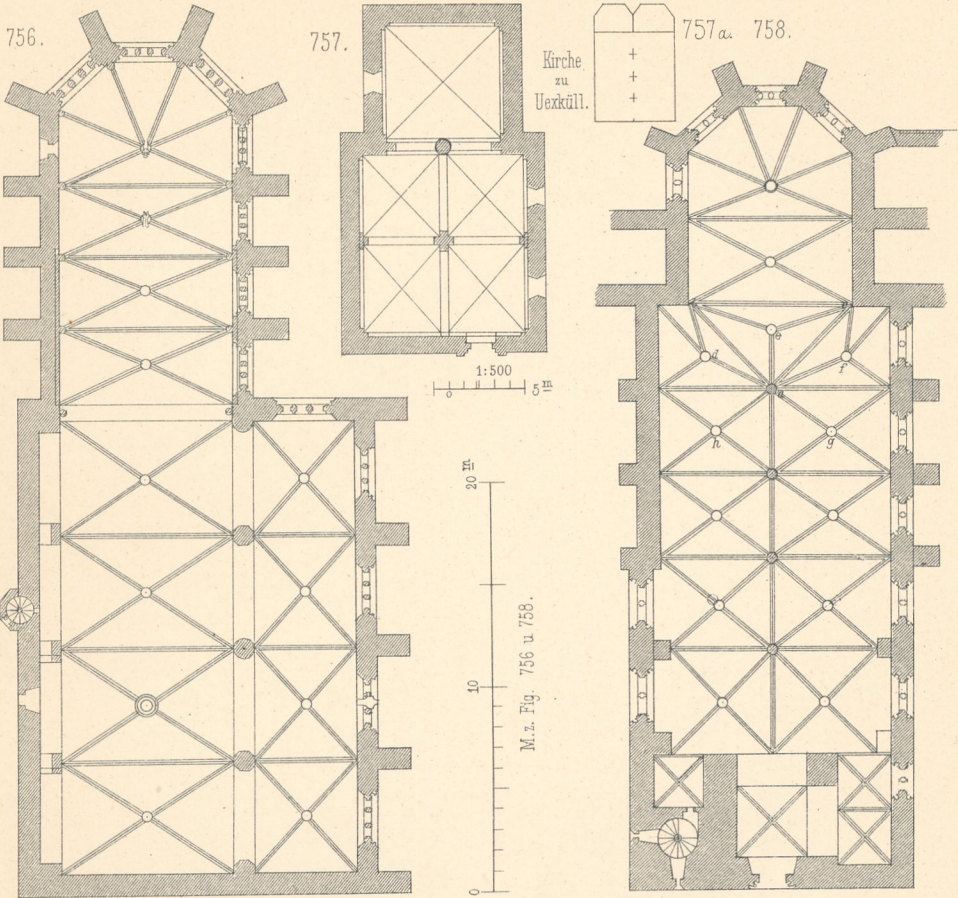
Klosterkirche zu Bornhofen.
