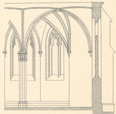
Schnitt zu Fig. 758.
