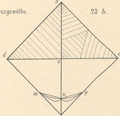
Gewölbe ohne Ueberhöhung u. Busung.
