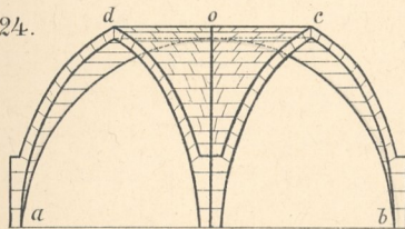
Gewölbe ohne Ueberhöhung u. Busung.
