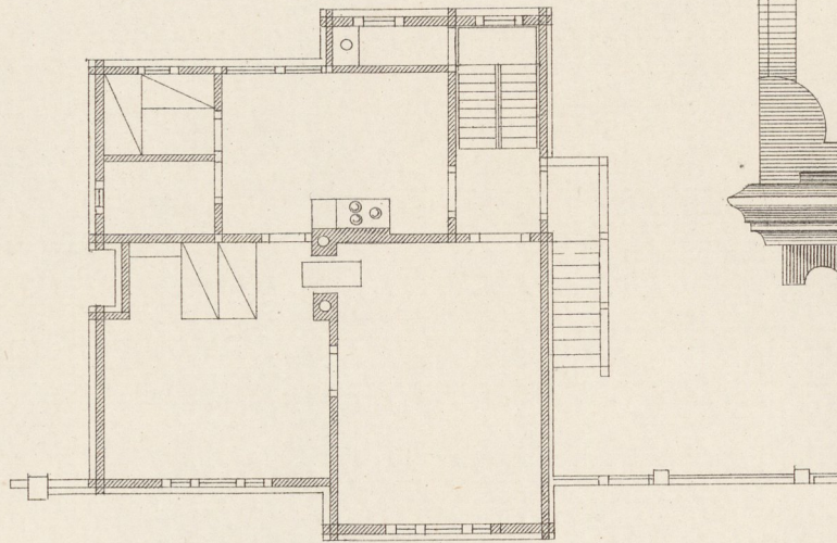
Grundriss
