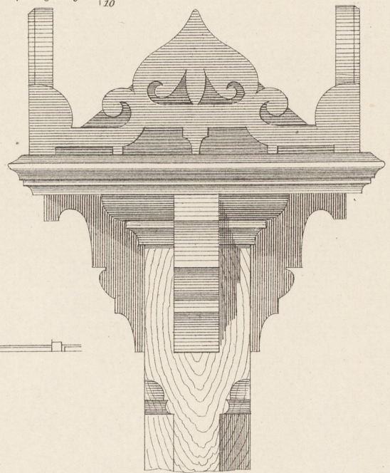
Thorsäulenkapf
