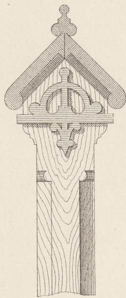
Thürsäulenkapf
