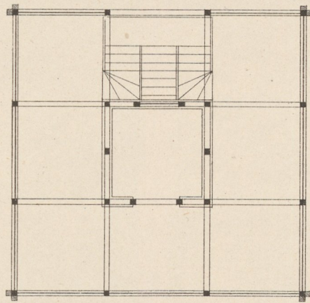
Grundriss.
