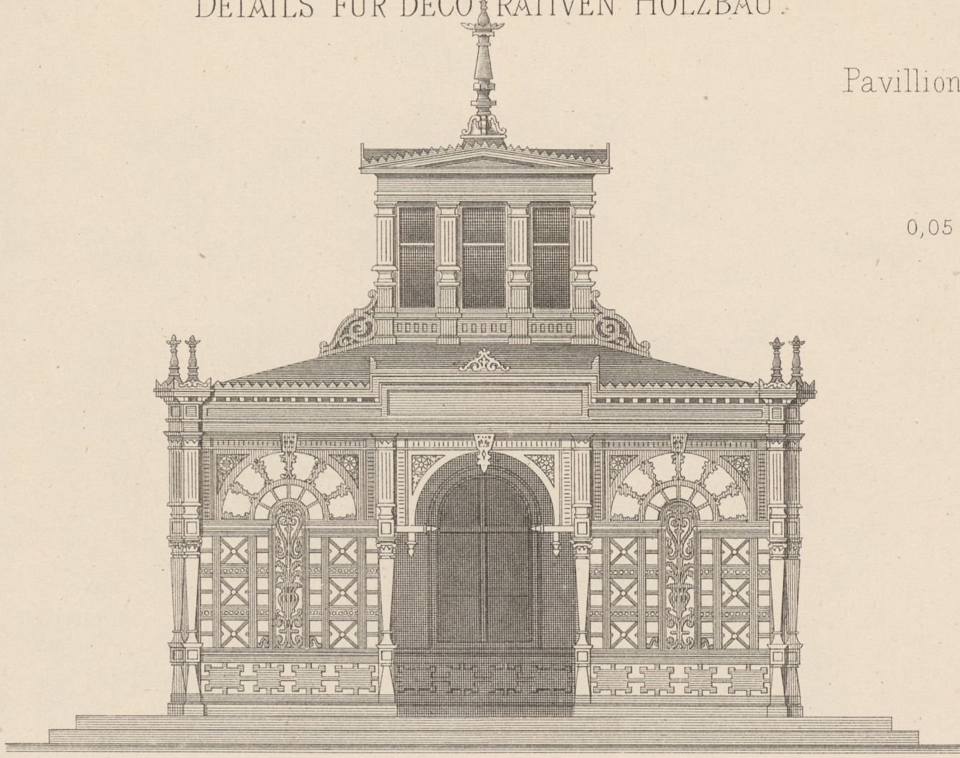
Façade.
