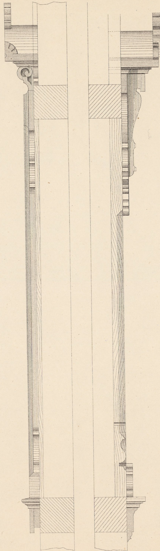
Fenster Einfaltungen 0,1 natürlicher Grösse:
