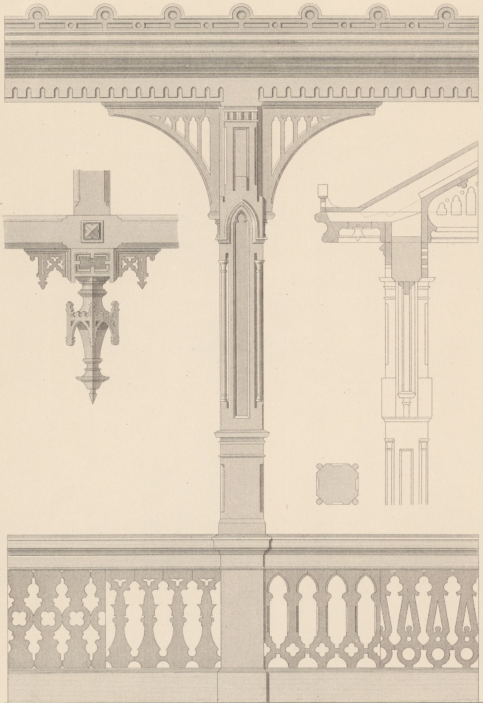
Theile einer bedekten Halle und Hängesäule
