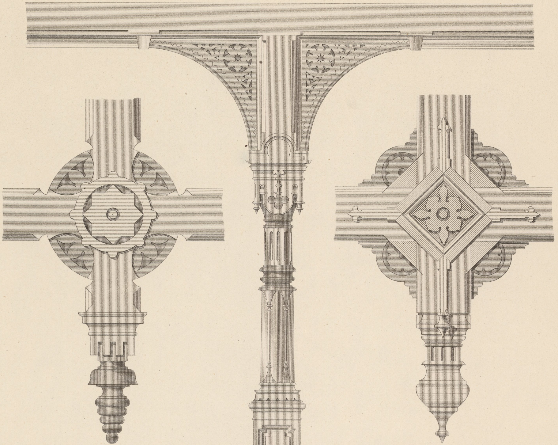
Decoration für Hängesäulen und — — Kehlbalcken an Dachgiebeln
