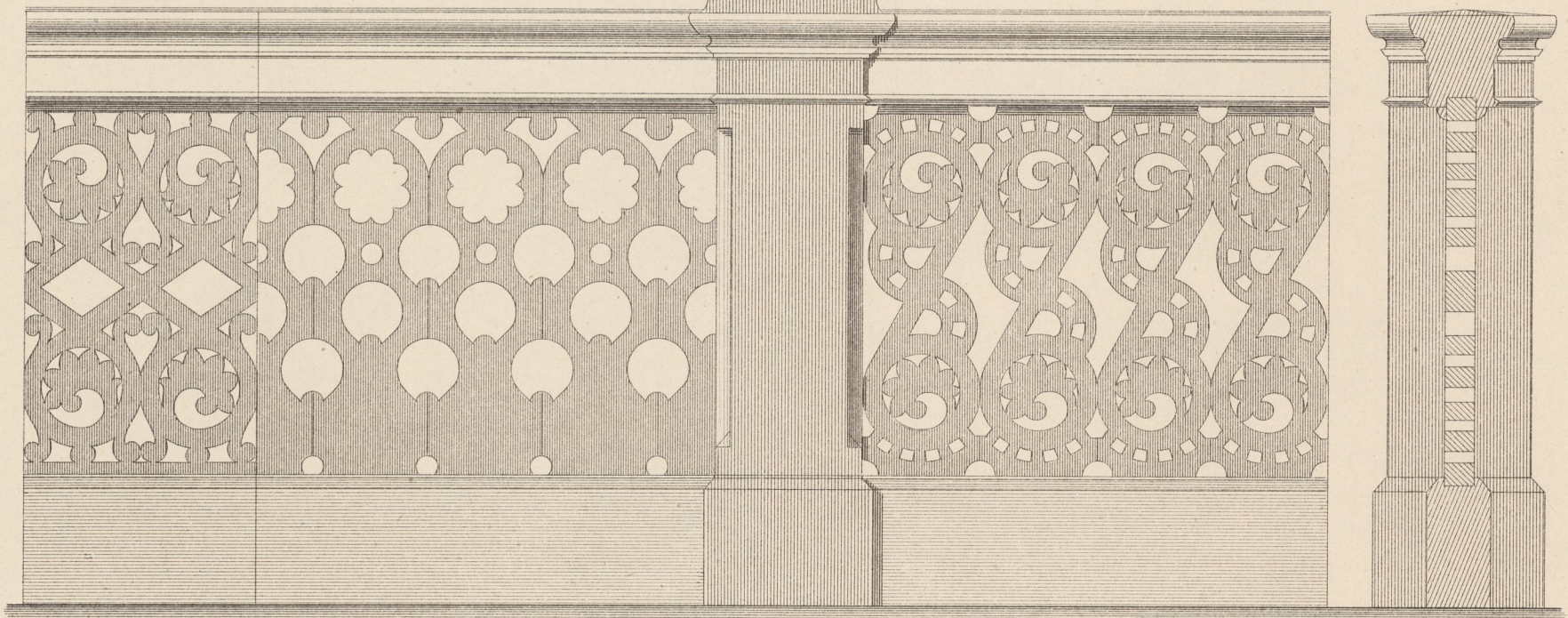
Dachpfette, Säule und Geländer für eine Veranda.
