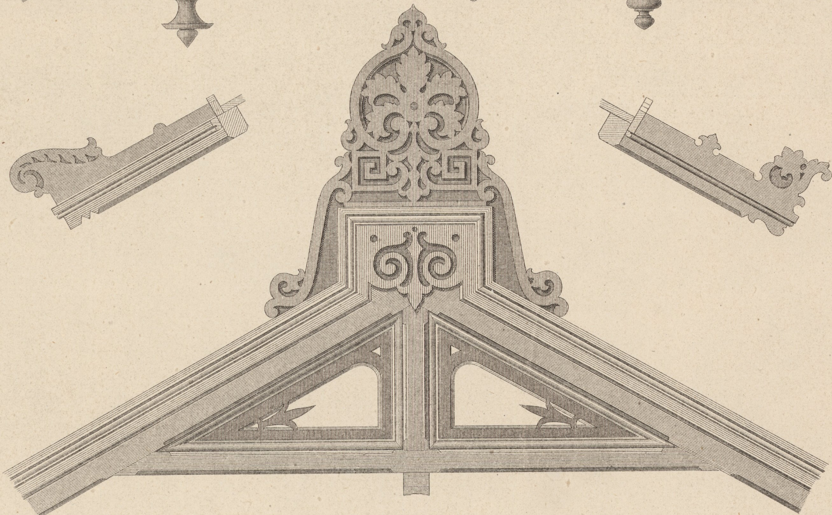
Decoration von Giebelconstructionen.
