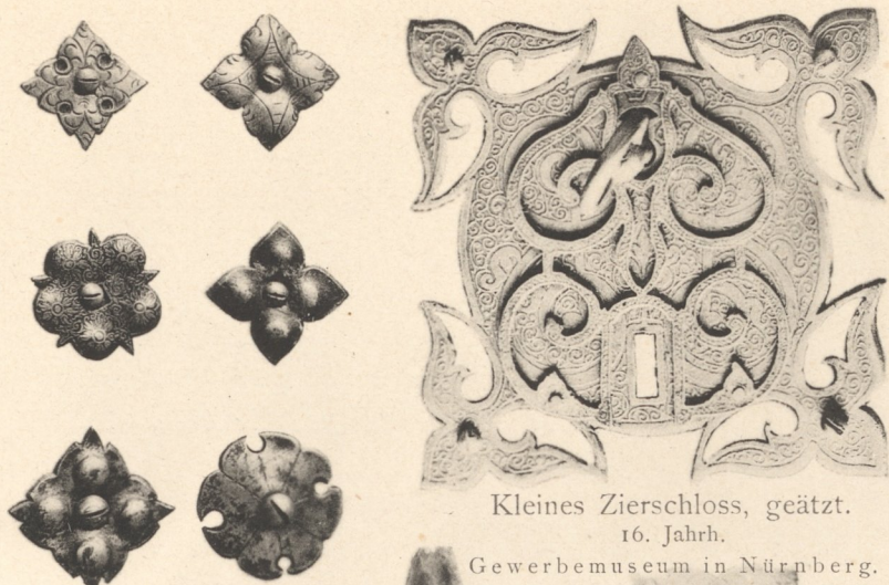
Getriebene Rosetten für Thür- und Fensterbeschläge. 16. u. 17. Jahrh. Germ. Museum in Nürnberg.
