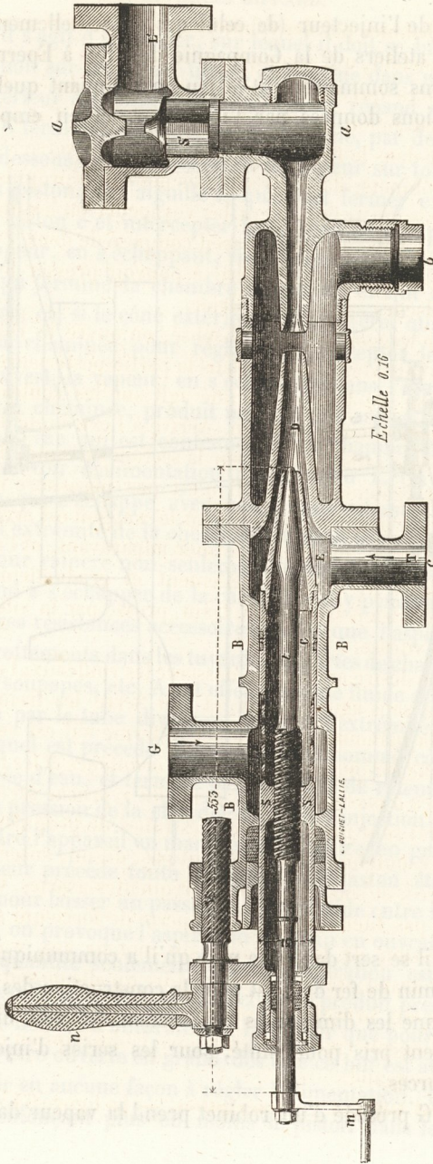
Fig. 645. — Appareil Giffard. Coupe.
