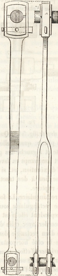
543. — Bielle à fourche.
