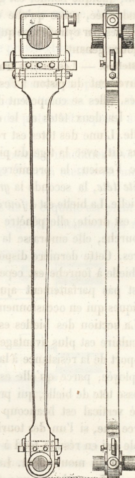
544. — Bielle droite.
