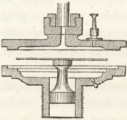
Fig. 511. — Manomètre Galy-Cazalat.
