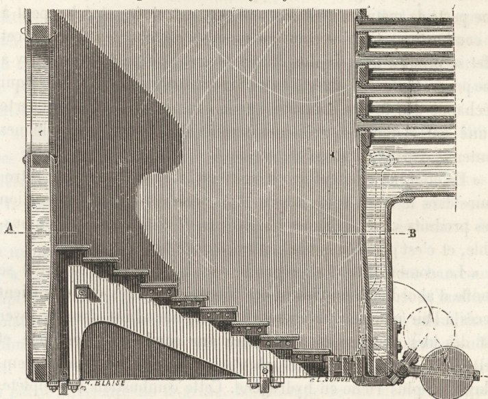
Fig. 498. — Coupe d'un foyer à grille Chobrzynsky.
