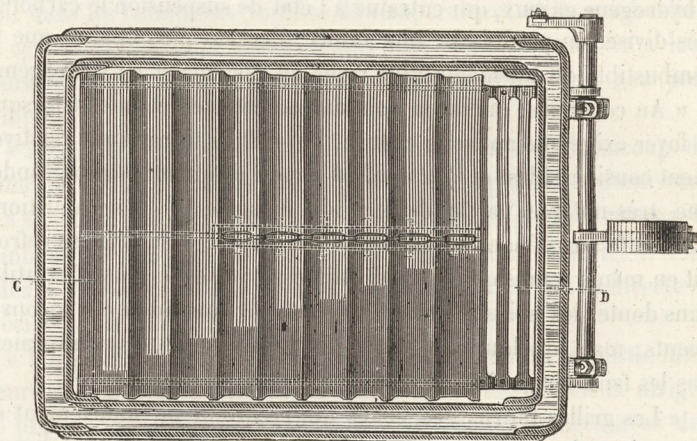
Fig. 499. — Plan d'un foyer à grille Chobrzynsky.
