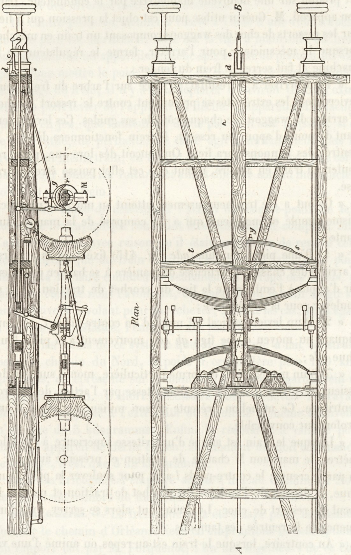
Fig. 415. — Frein automoteur Guérin.
