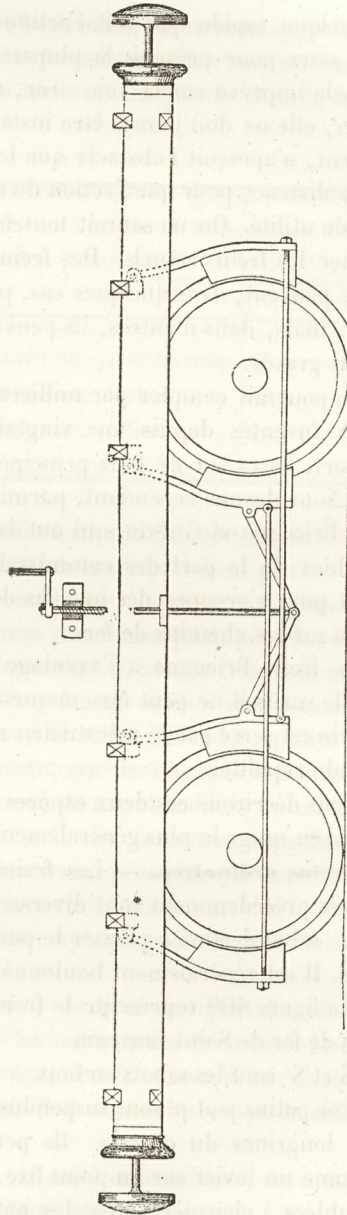
Fig. 410. — Ancien frein de Versailles (rive gauche).
