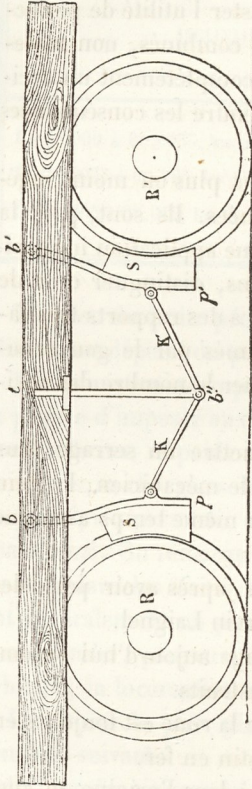
Fig. 409. — Ancien frein du chemin de Saint-Germain.
