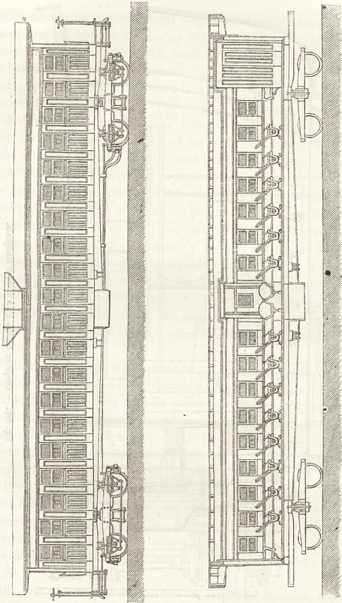
Fig. 407. — Élévation et coupe longitudinale d'un waggon américain.
