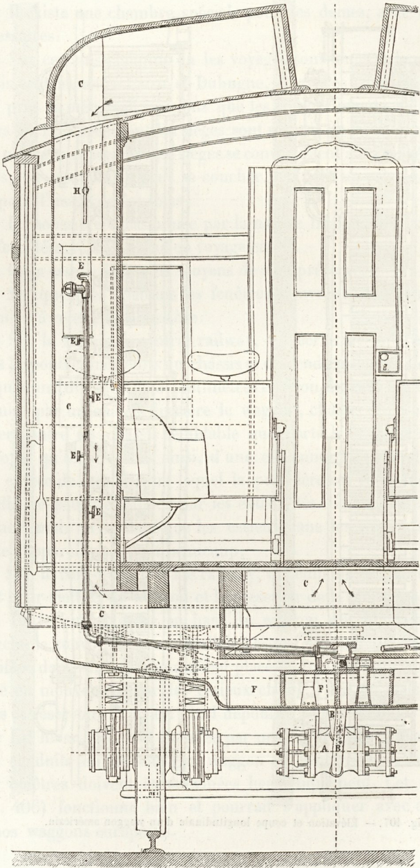
Fig. 406. — Coupe en travers d'un wagon américain.
