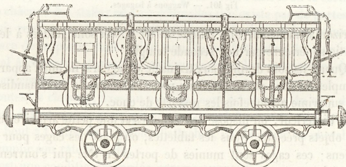
Fig. 405. — Coupe d'une voiture de 1 re classe.
