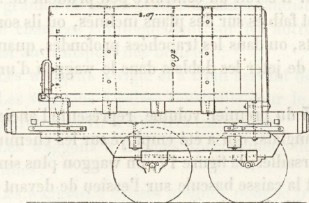
Fig. 598. — Waggon anglais grand modèle.
