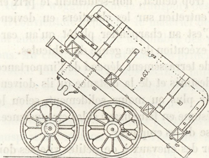
Fig. 597. — Waggon anglais petit modèle.
