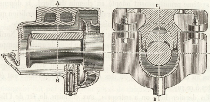
Fig. 581. — Boîte à huile de Dietz, à fusée immergente.
