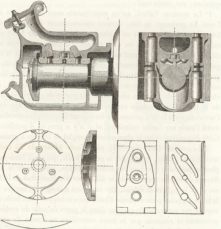
Fig. 582. — Autre boîte à huile.
