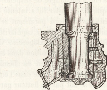
Fig. 378 b. — Boîte à huile à levier à contre-poids.
