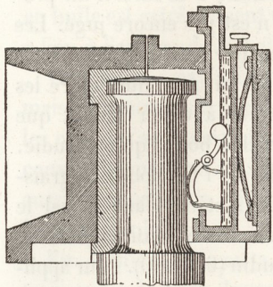
Fig. 378 b. — Boîte à huile à levier à contre-poids.
