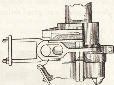
Fig. 379. — Boîtes à graisse et à huile du chemin de fer du Nord.
