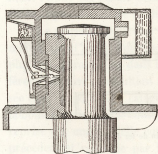
Fig. 378 a. — Boîte à huile à siphon.
