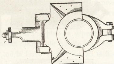
Fig. 379. — Boîtes à graisse et à huile du chemin de fer du Nord.
