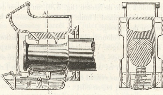
Fig. 576. — Boîte du chemin de Tours à Nantes.
