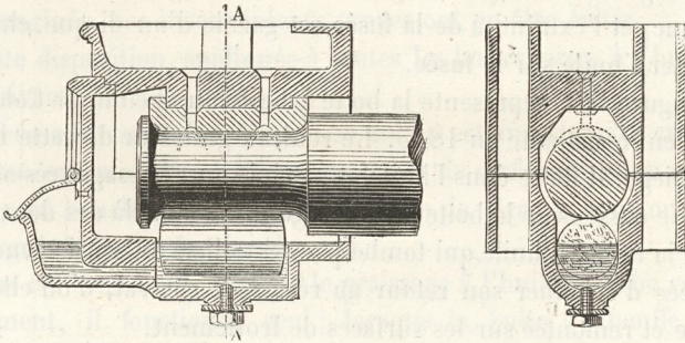
Fig. 575. — Boîte du chemin de Co'logne à Minden.
