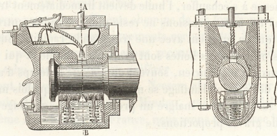
Fig. 577. — Boîte Neesen (Oppeneau).
