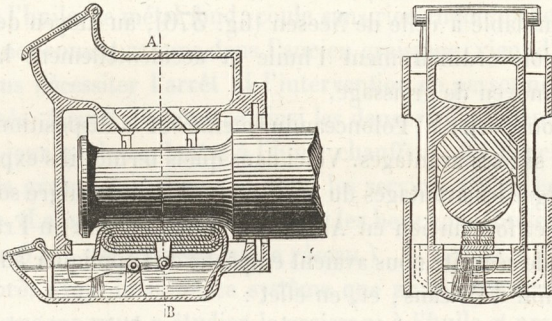
Fig. 576. — Boîte du chemin de Tours à Nantes.
