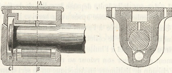
Fig. 574. — Boîte Winans, de Baltimore.
