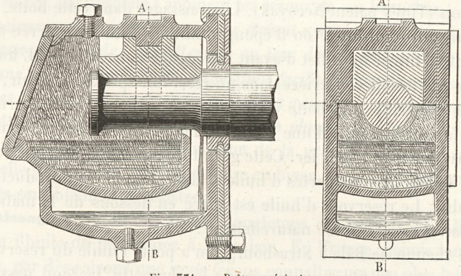
Fig. 571. — Boîte américaine.
