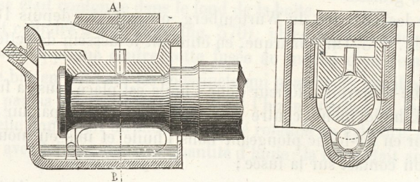
Fig. 375. — Boîte wurtembergeoise.
