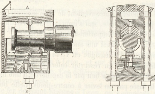
Fig. 572. — Boîte badoise importée par M. Lechatelier.
