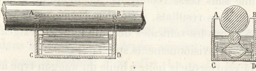
Fig. 570. — Poitè de Séguin ainé (chemin de Saint-Étienne).
