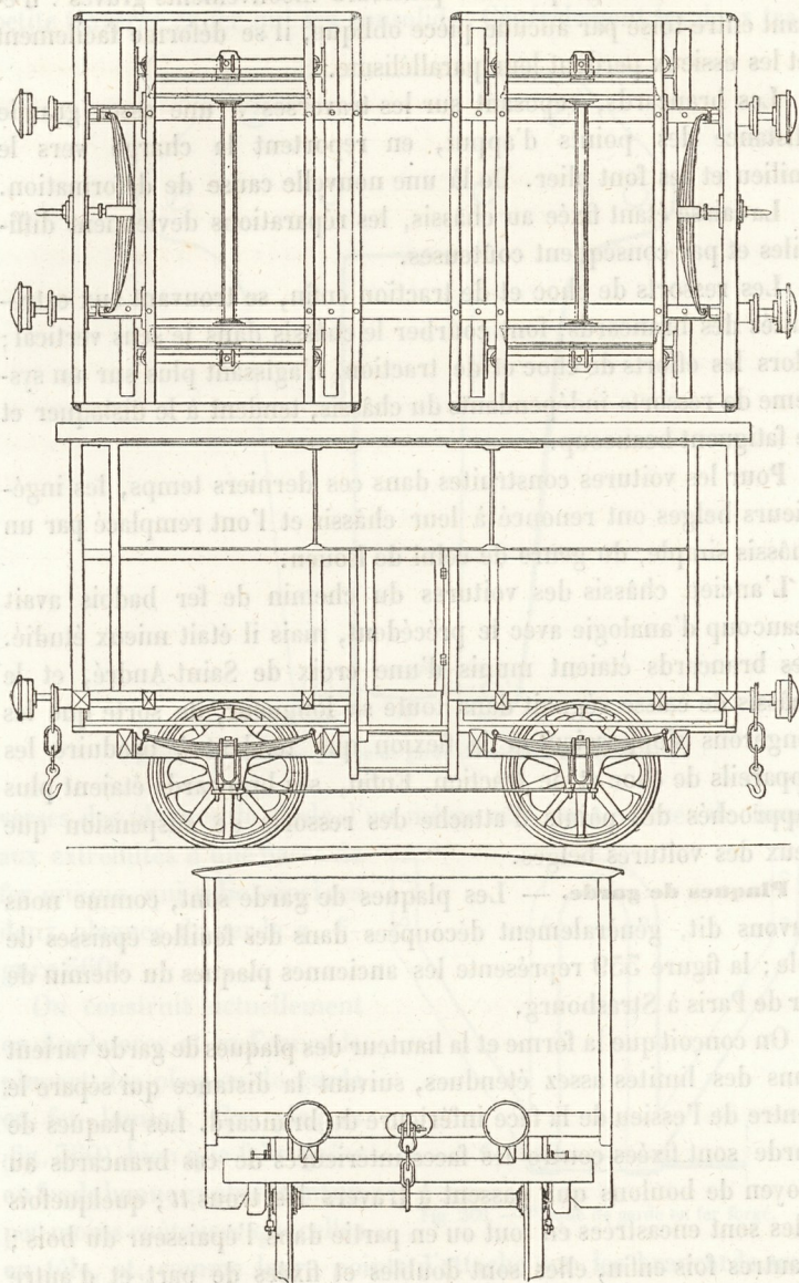
Fig. 558. — Châssis de voitures belges.
