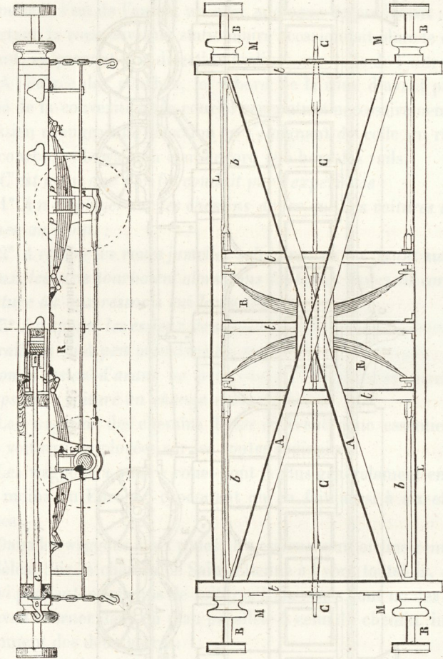
Fig. 555. — Châssis du chemin de fer de Rouen.
