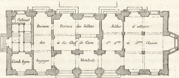
Fig. 531. — Station du second ordre des chemins de fer badois.
