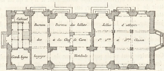
Fig. 531. — Station du second ordre des chemins de fer badois.
