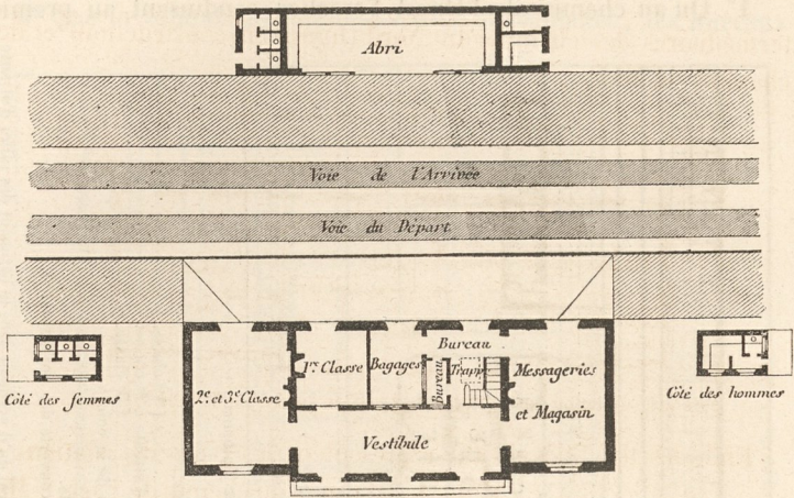
Fig. 504. — Station intermédiaire du chemin de Chartres.
