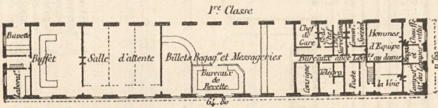
Fig. 506. — Station intermédiaire du chemin du Midi.
