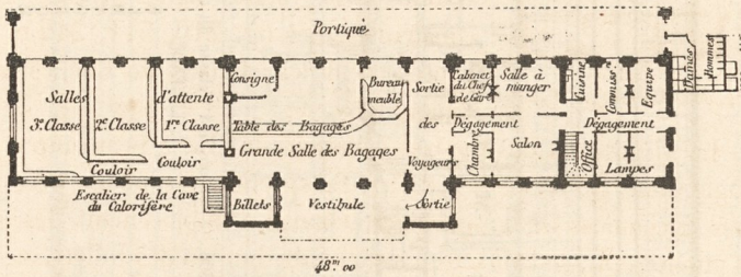
Fig. 505. — Station intermédiaire de 1re classe du chemin du Nord.
