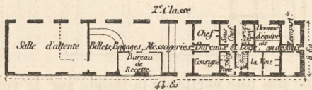
Fig. 507. — Station intermédiaire du chemin du Midi.
