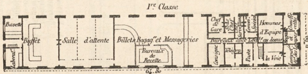
Fig. 506. — Station intermédiaire du chemin du Midi.
