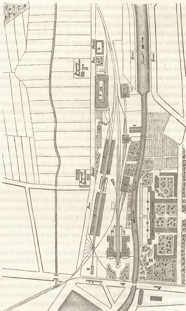
Fig. 282. — Plan de la gare du chemin de Berlin à Hambourg, à Bertin. (Voir la légende, p. 69.)
