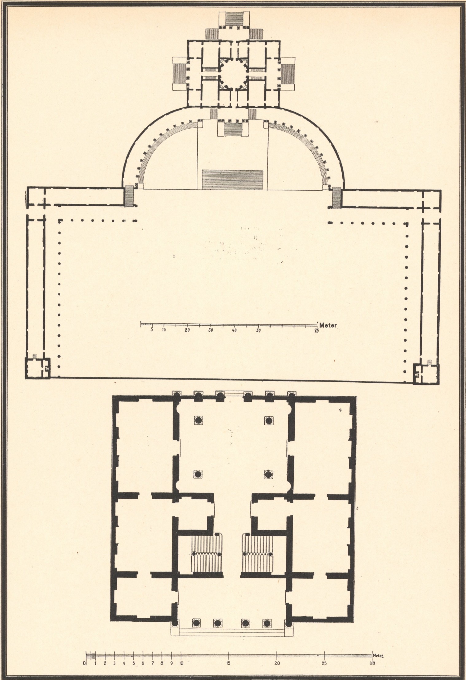
OBEN: VILLA TRISSINO IN MELEDO UNTEN: PALAZZO ANTONINI IN UDINE
