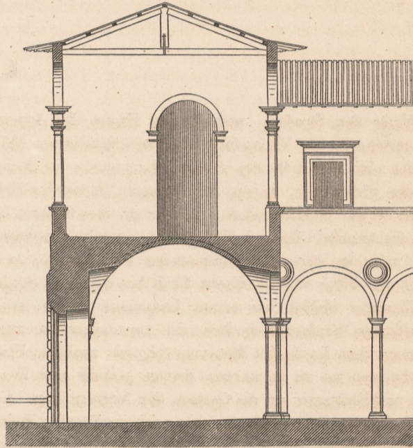
No. 3. Durchschnitt durch die Hofhalle der Villa zu S. Giustino.
