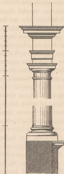
Nr. 4. Details zu den oberen Arcaden der Hofhalle der Villa zu S. Giustino.
