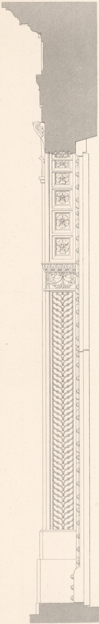
Schnitt.
