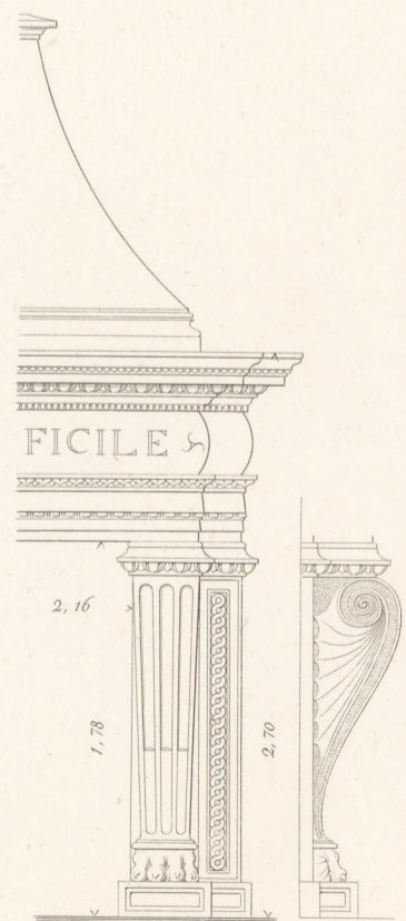
Camin in der Casa Deli.
