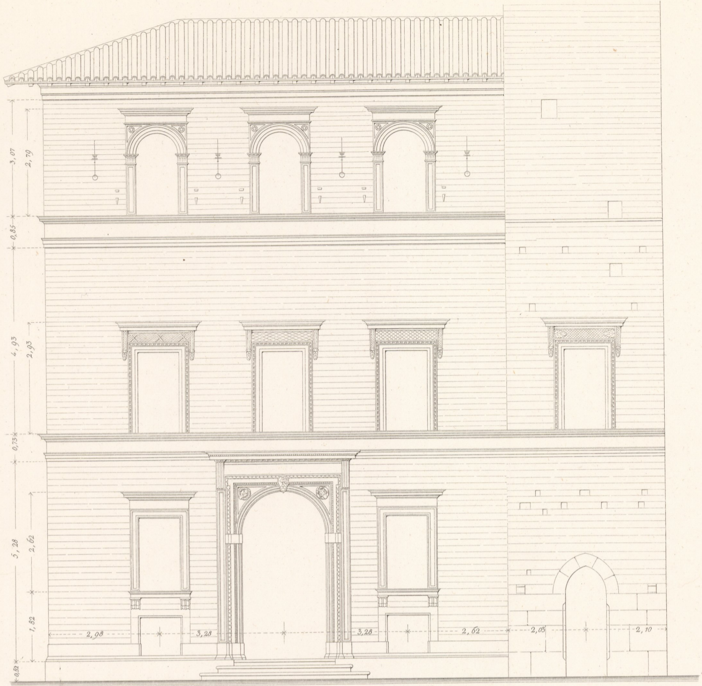
Vorder - Ansicht. Casa Deli zu Foligno.
