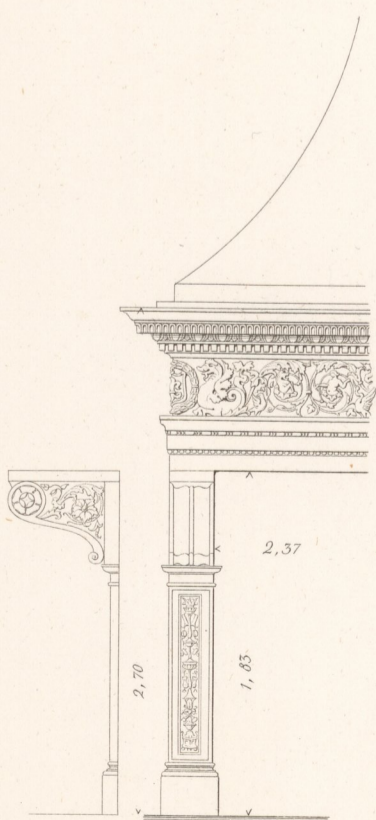
Kamin im Pal. Comunale.
