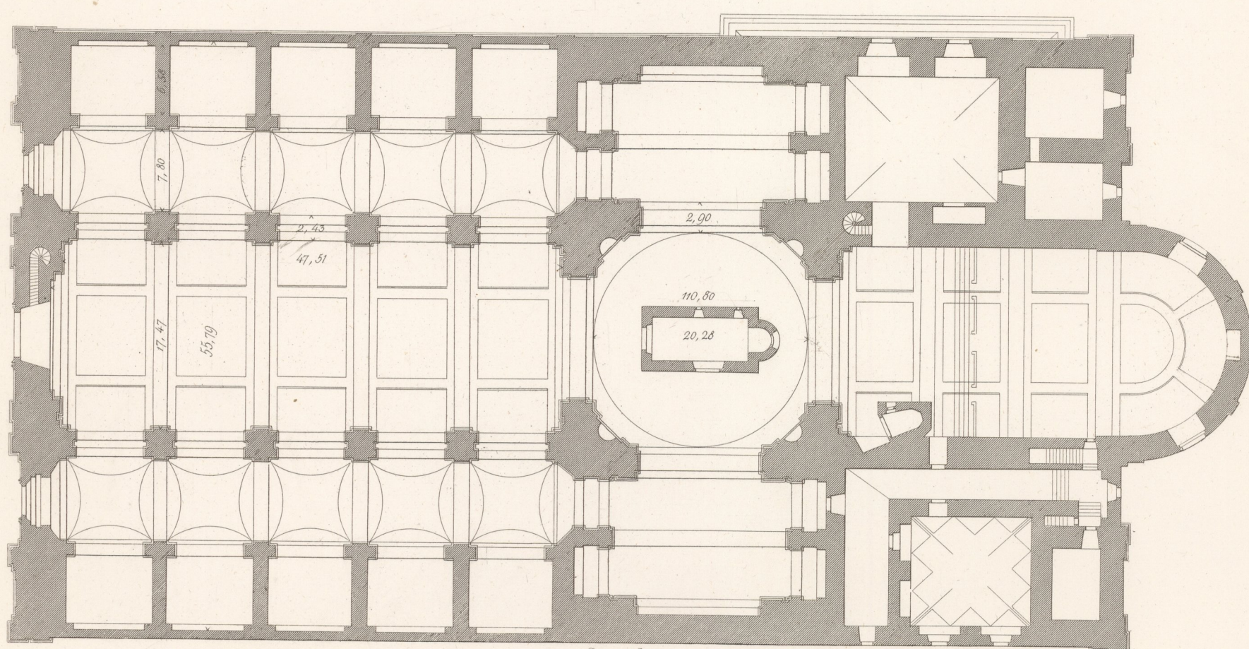
Grundriss.
