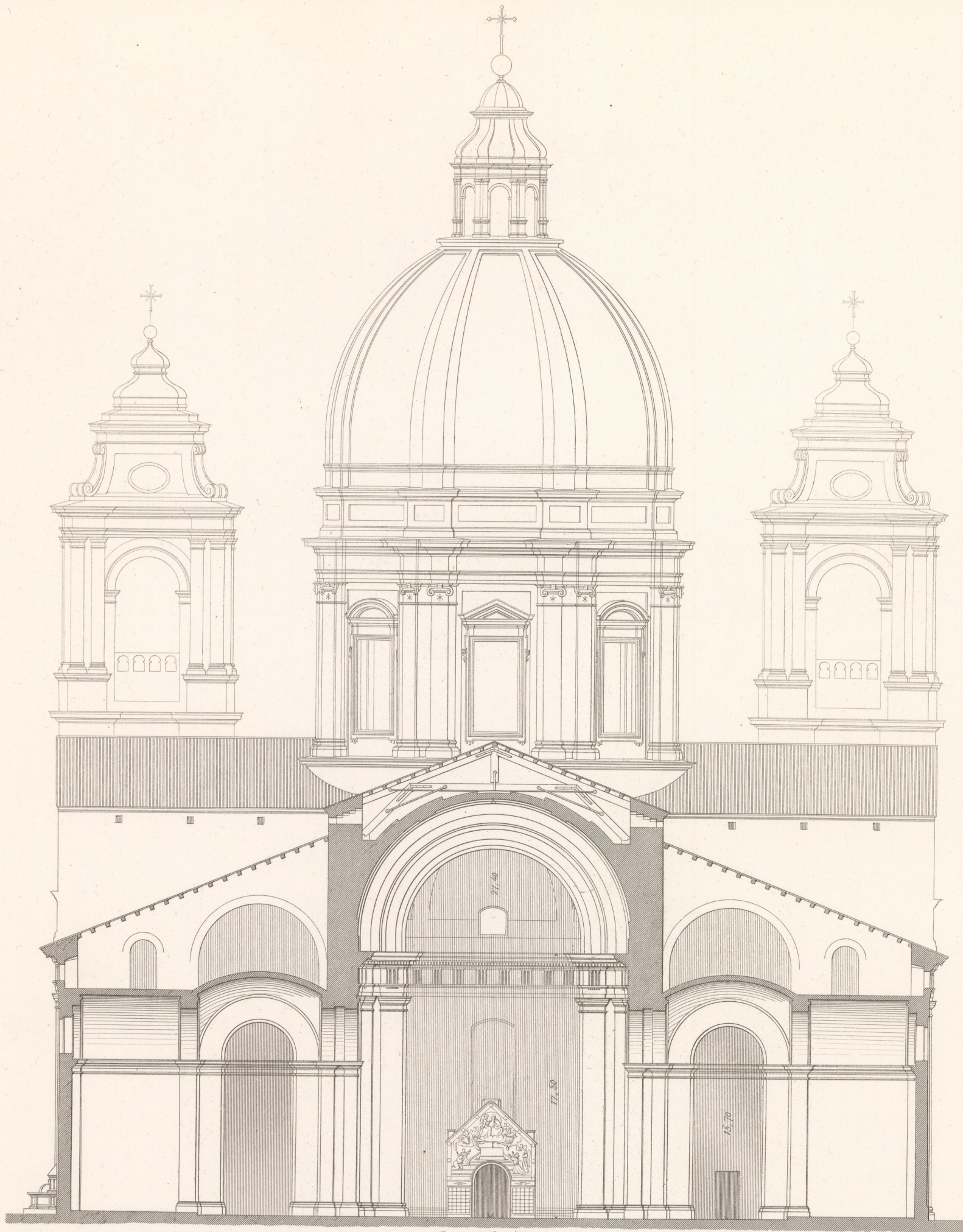
Querschnitt.
