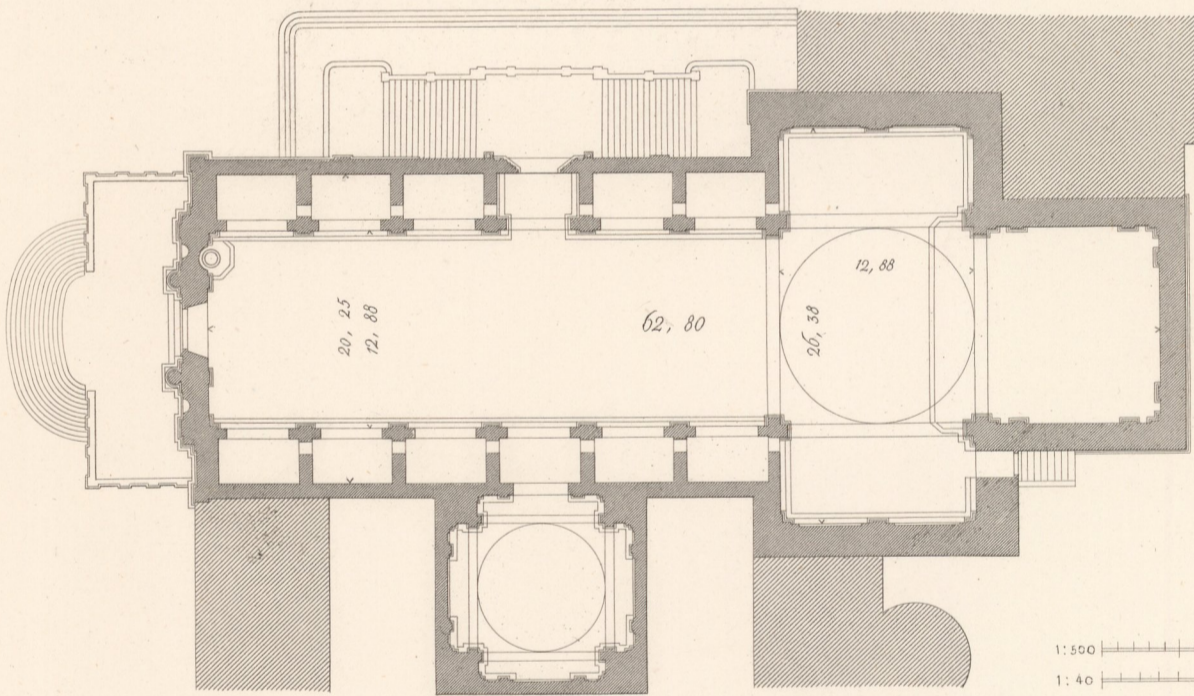
Grundriss.
