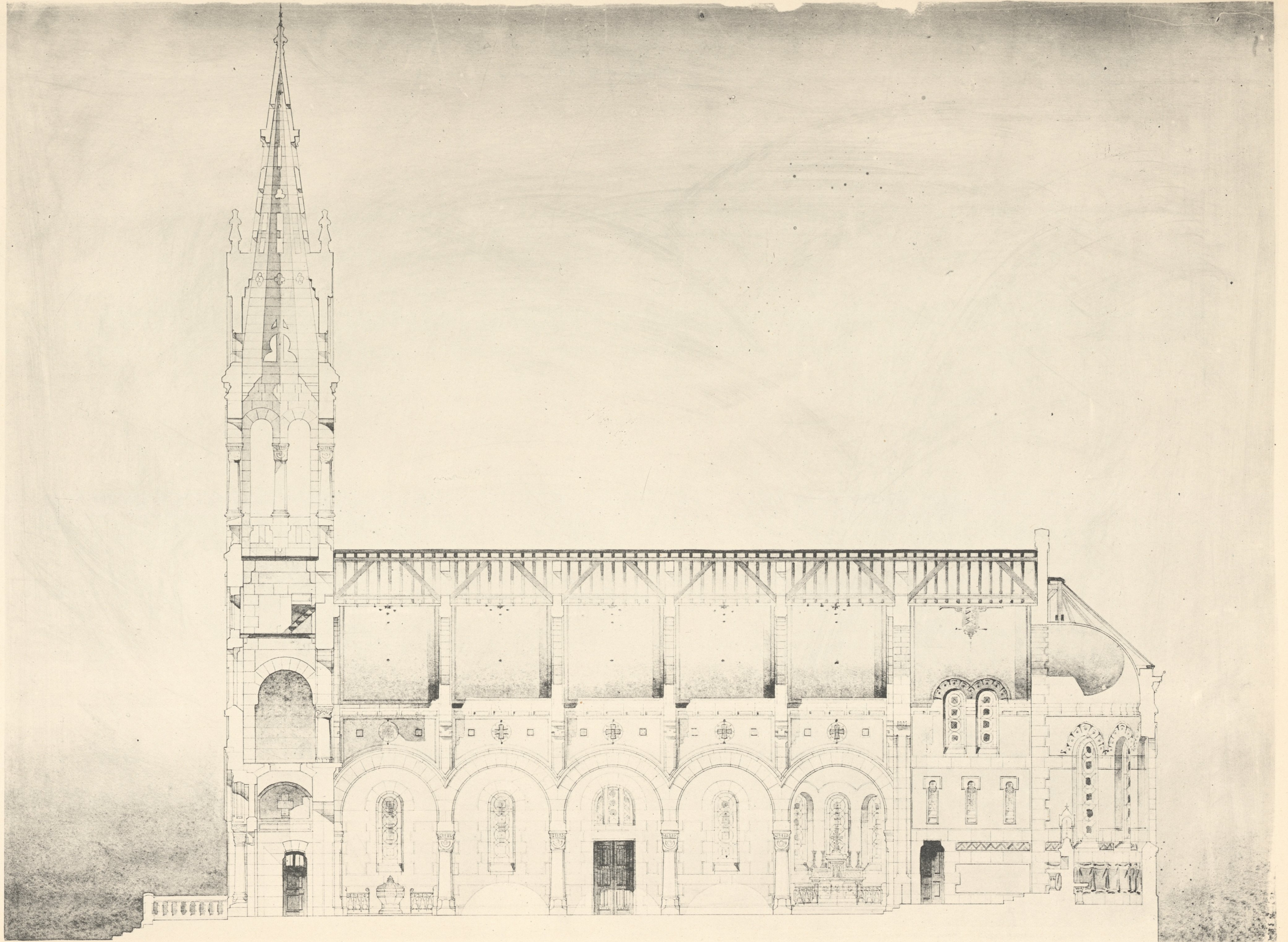
COUPE LONGITUDINALE LUCIEN-HENRI WOOG. - Église de Cesson (Saint-Brieuc).
