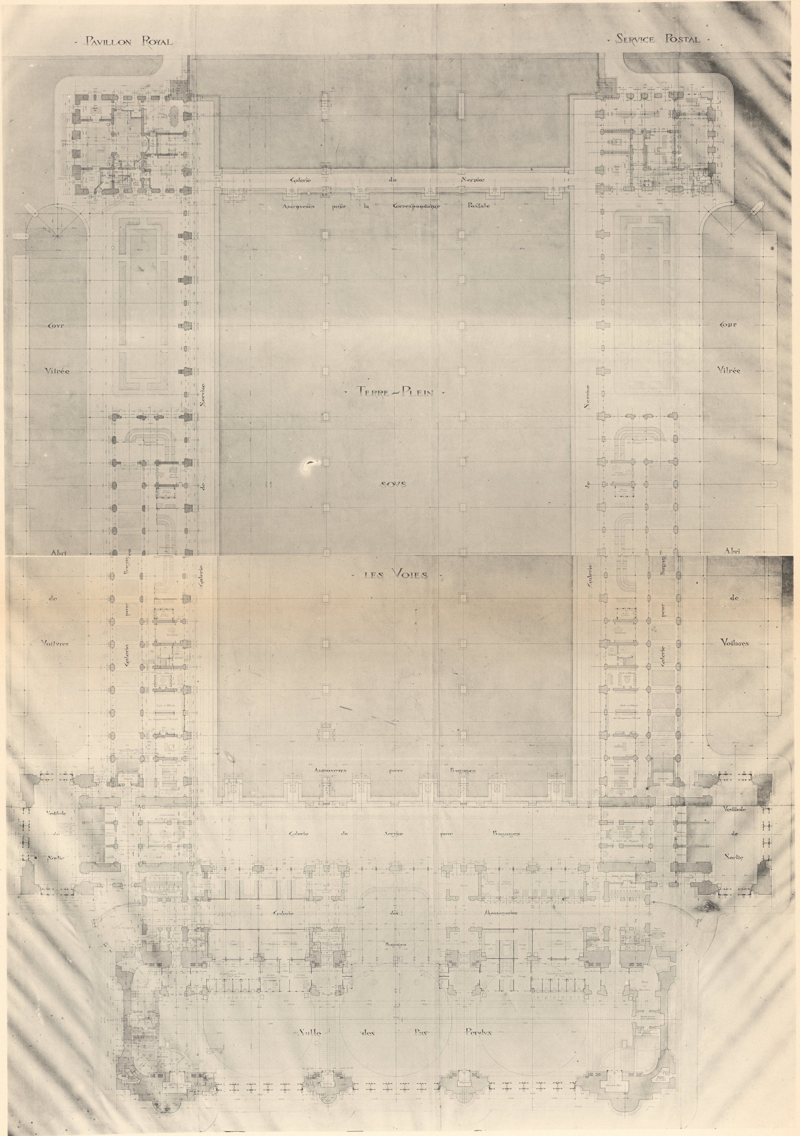
PLAN DU REZ-DE-CHAUSSÉE A.-A. MARCEL & L.-P. BLANC, - Gare centrale de Bucharest.
