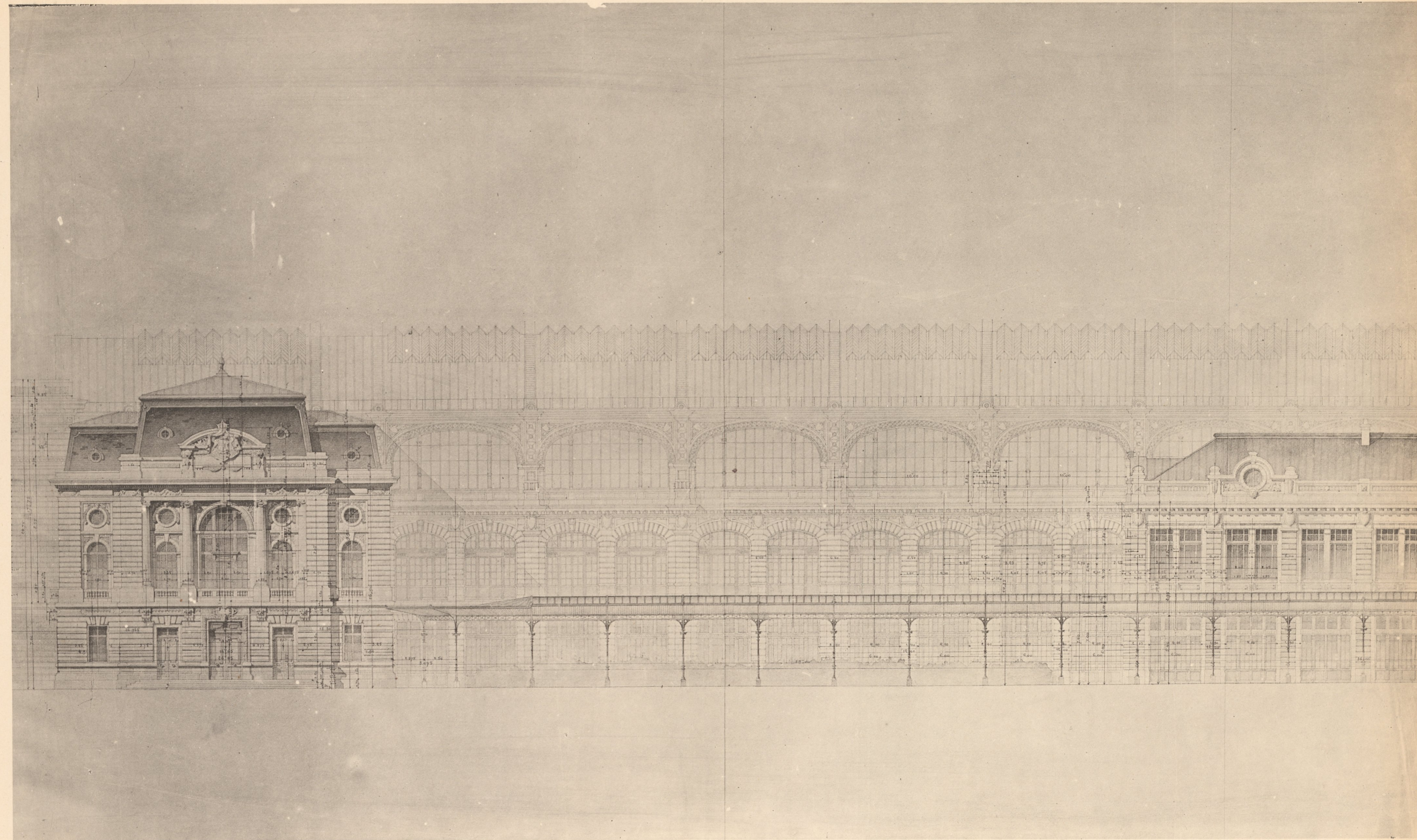
FAÇADE LATÉRALE A.-A. MARCEL & L.-P. BLANC. - Gare centrale de Bucharest.
