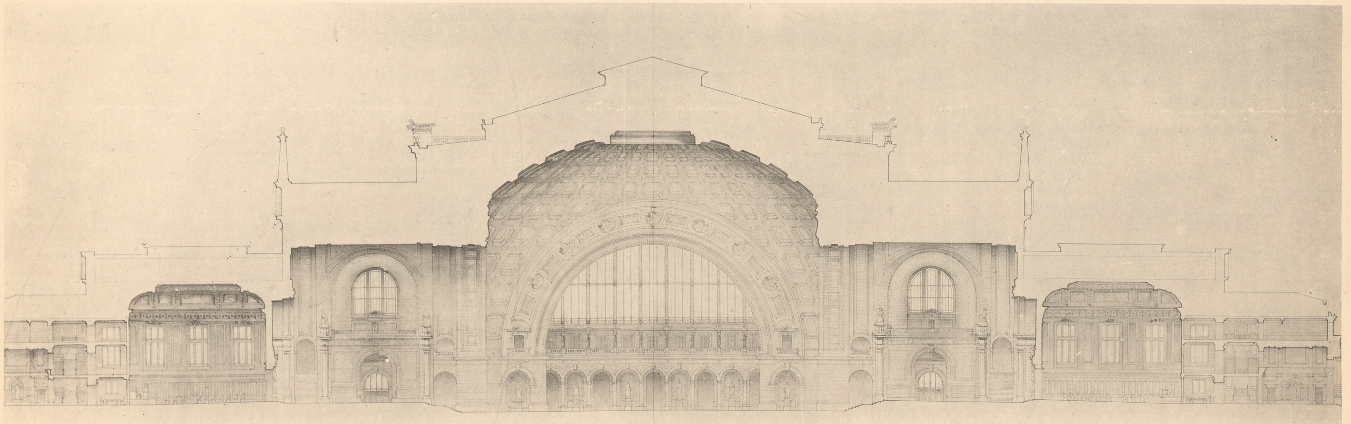
COUPE LONGITUDINALE
