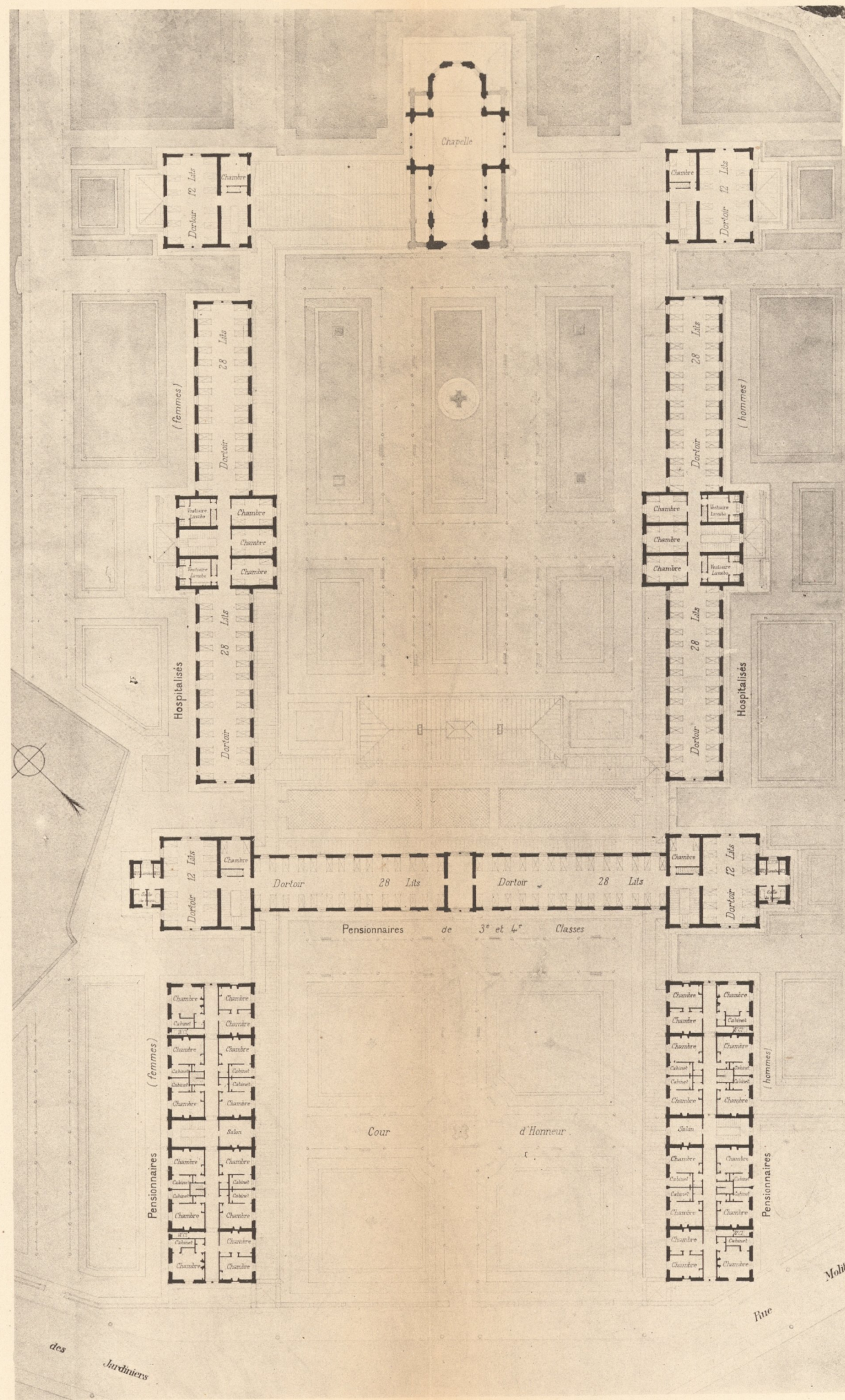
PLAN DU DEUXIÈME ÉTAGE
