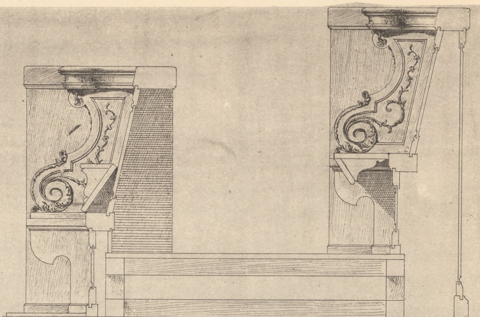
Coupe sur les Stalles.
