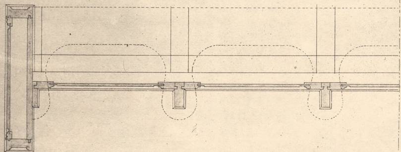
Plan au dessous des Sièges
