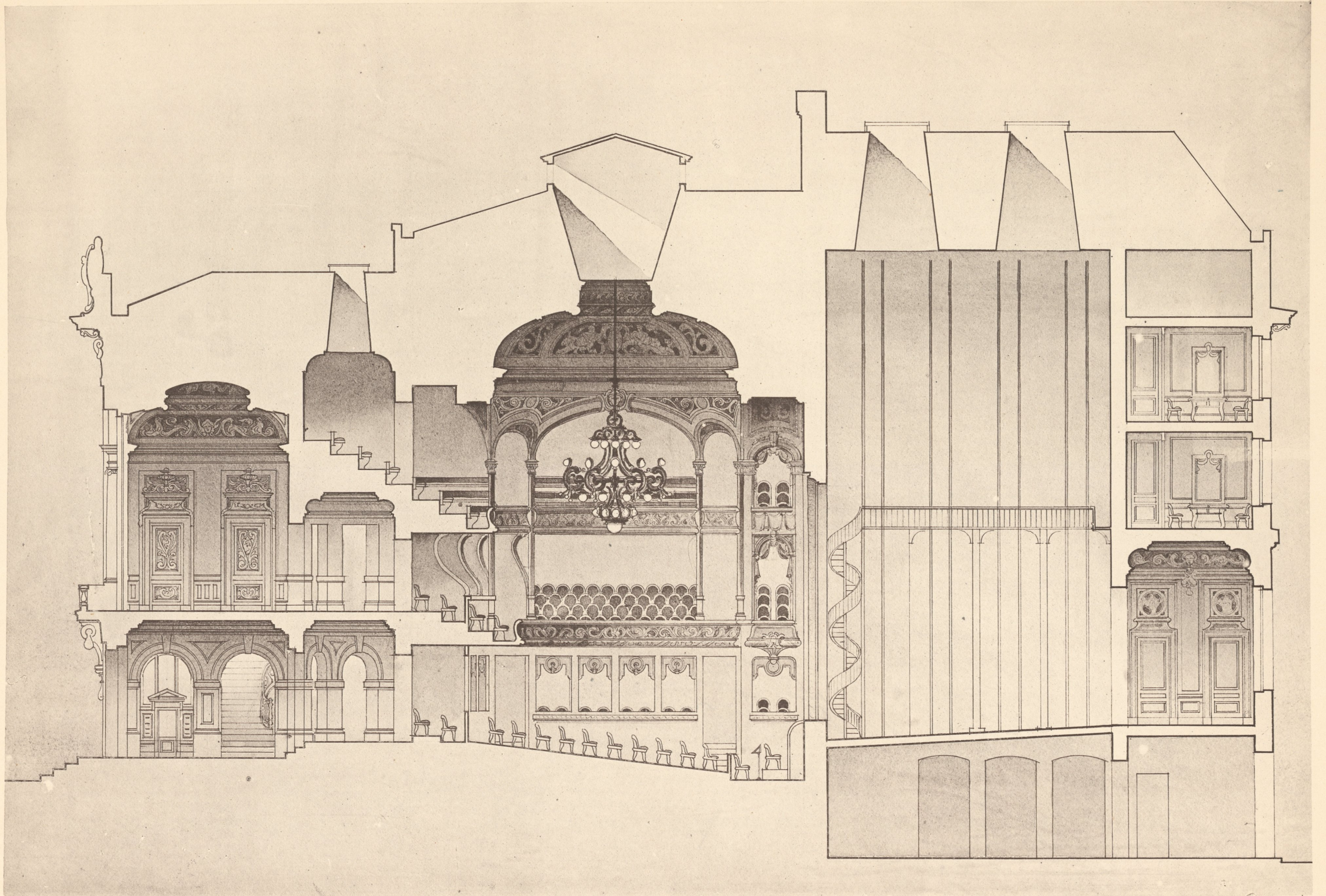
JOSEPH DUPONT. - Projet de Théâtre pour la ville de Noyon (Oise).
