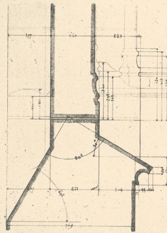
Coupe sur l'Axe de la Fenêtre
