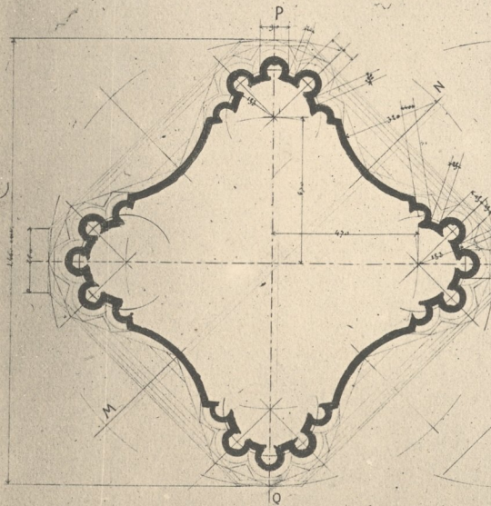
PILIER DE LA GRANDE NEF
