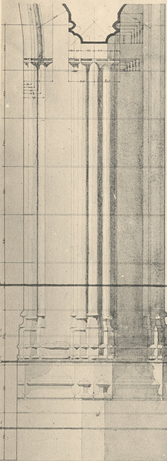
Coupe au Sommier de l'Arc
