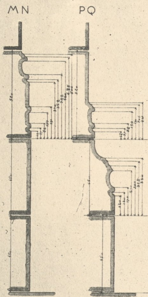
Coupes sur les Axes
