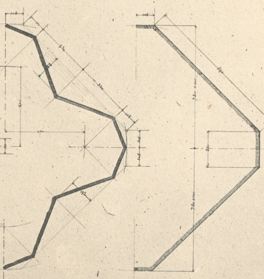
Plans suivant EF
