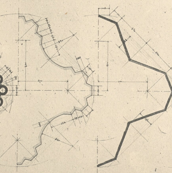
PILIER DE LA GRANDE NEF
