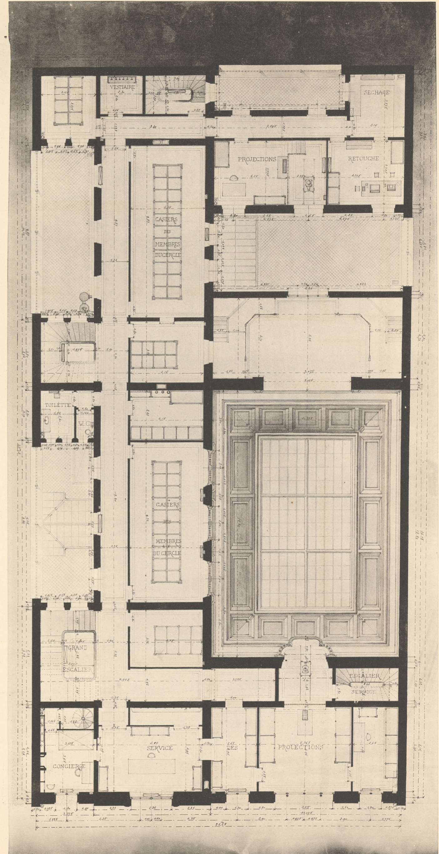
PLAN DE L'ENTRESOL.
