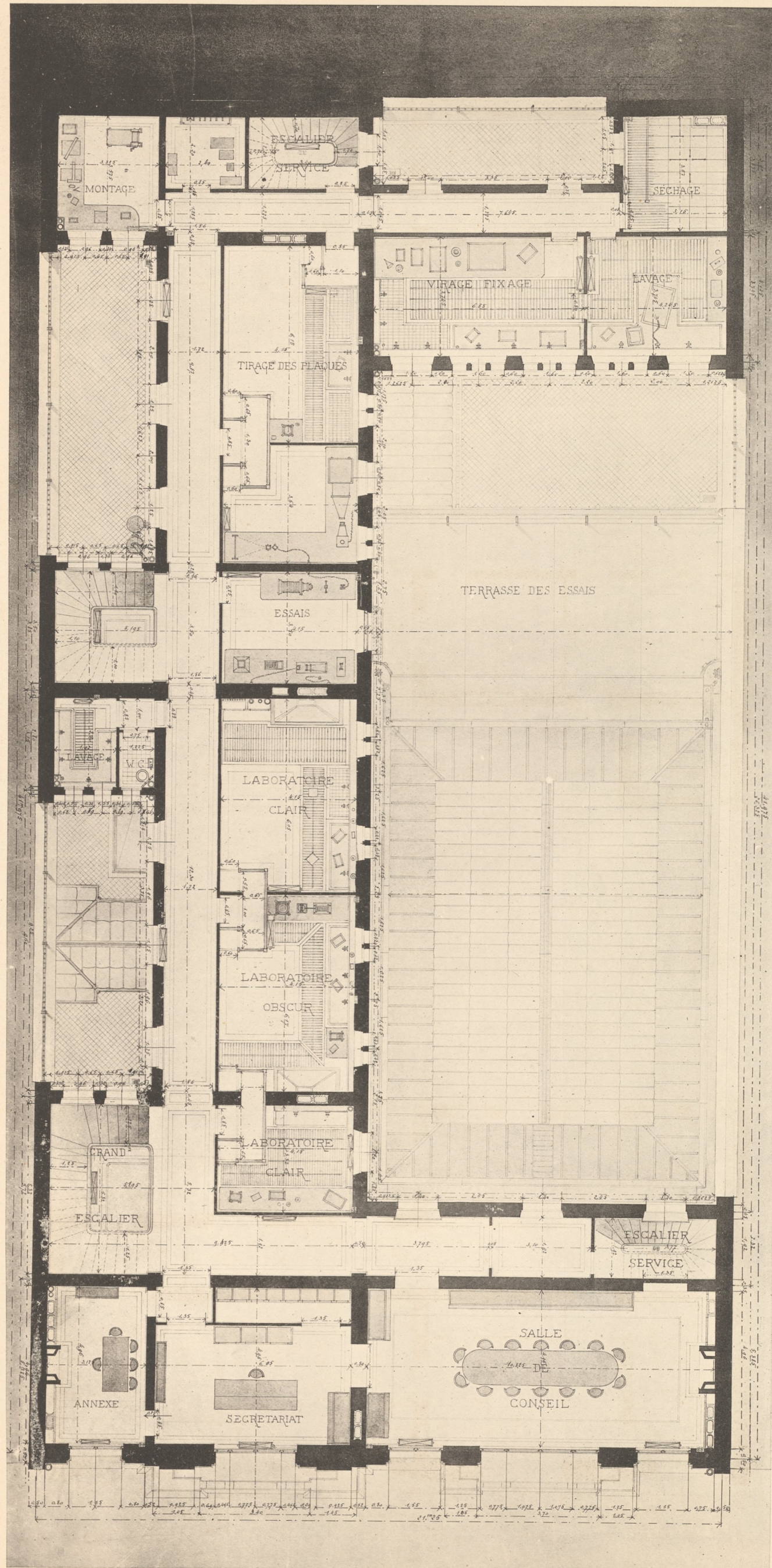
PLAN DU PREMIER ETAGE.
