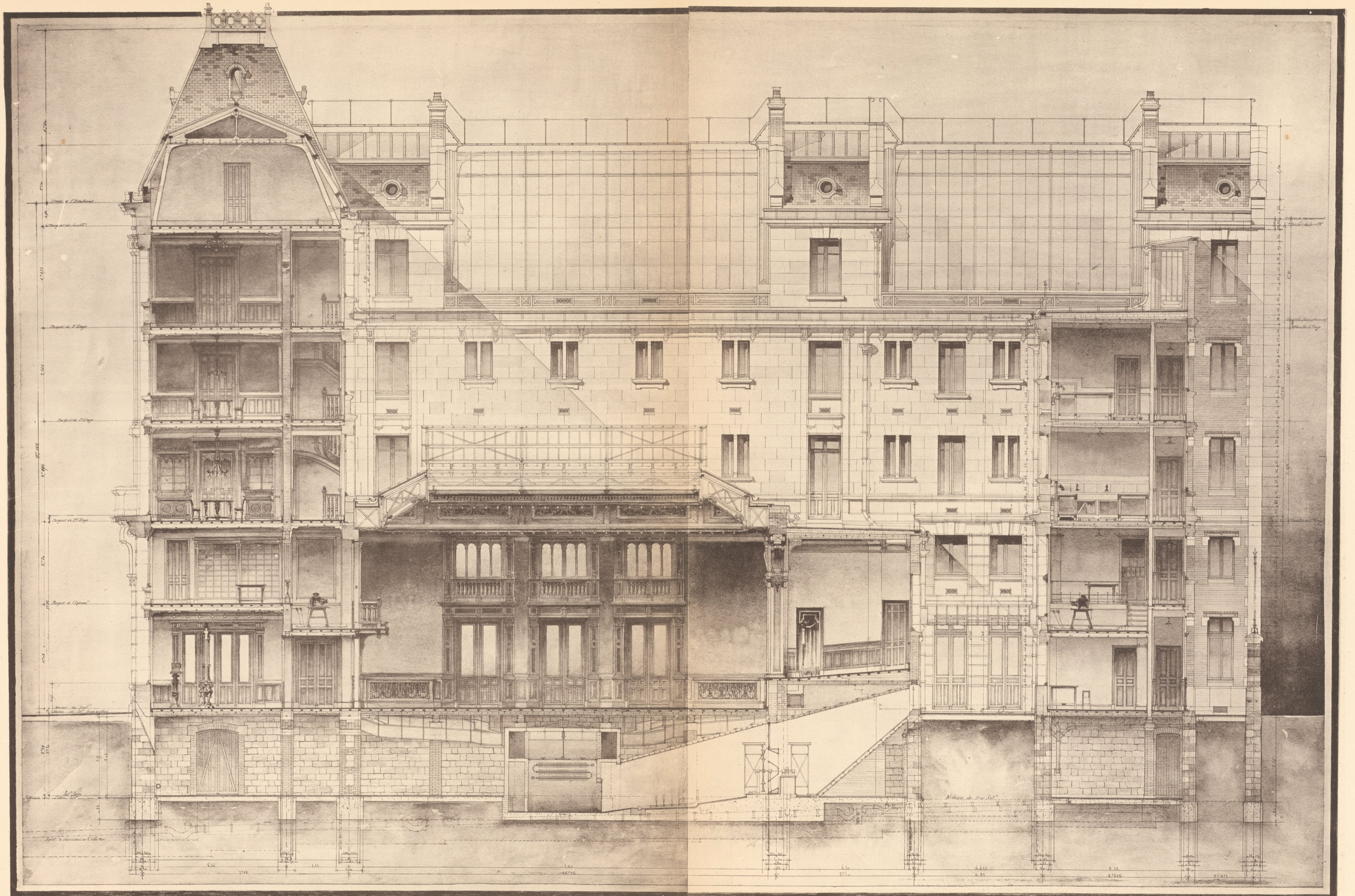
COUPE LONGITUDINALE P.-J. CLEMENT. - Un Photo-Club.
