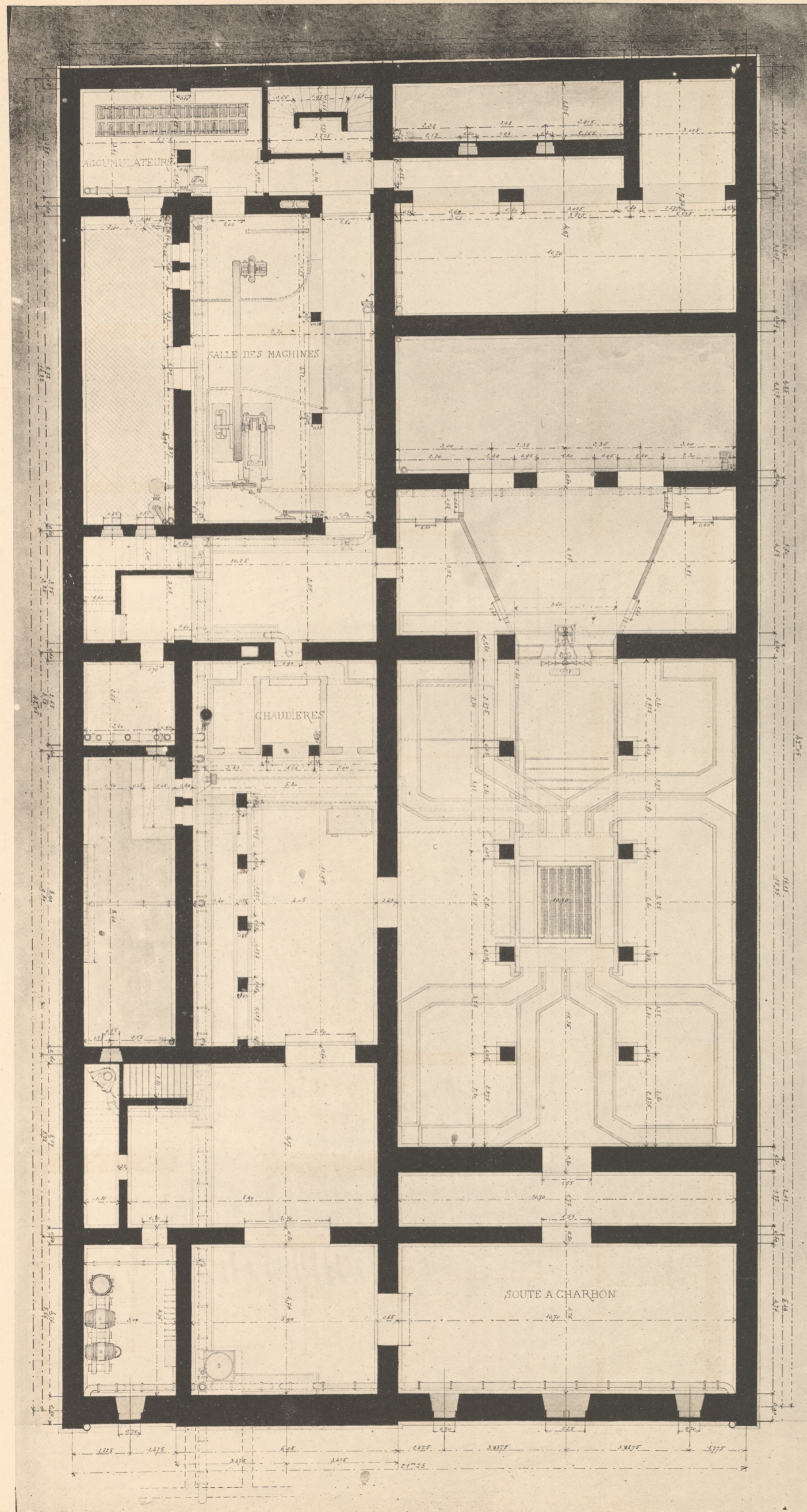
PLAN DU SOUS-SOL.
