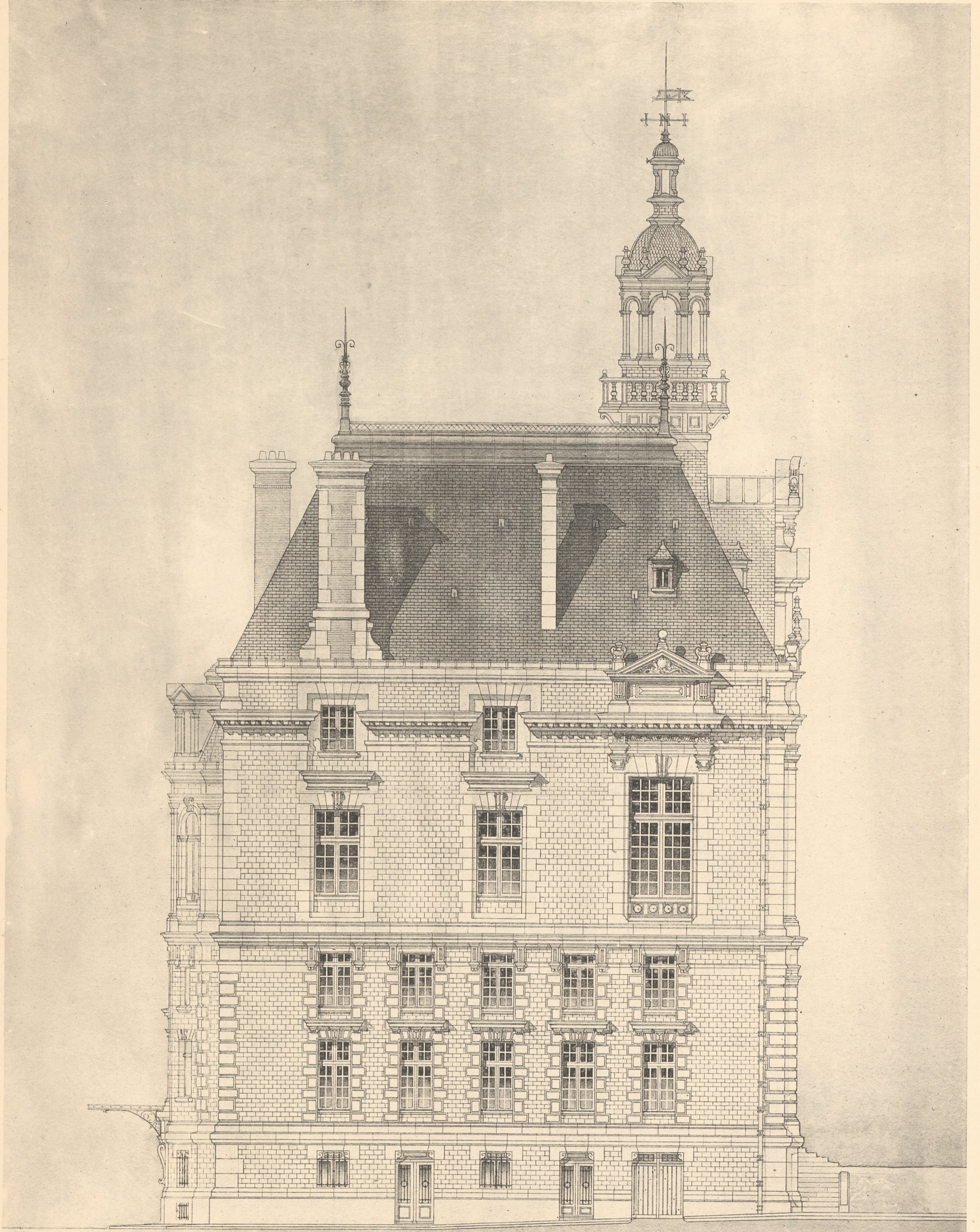
FAÇADE COTE DU MUR DE L'ECOLE POMPEE
