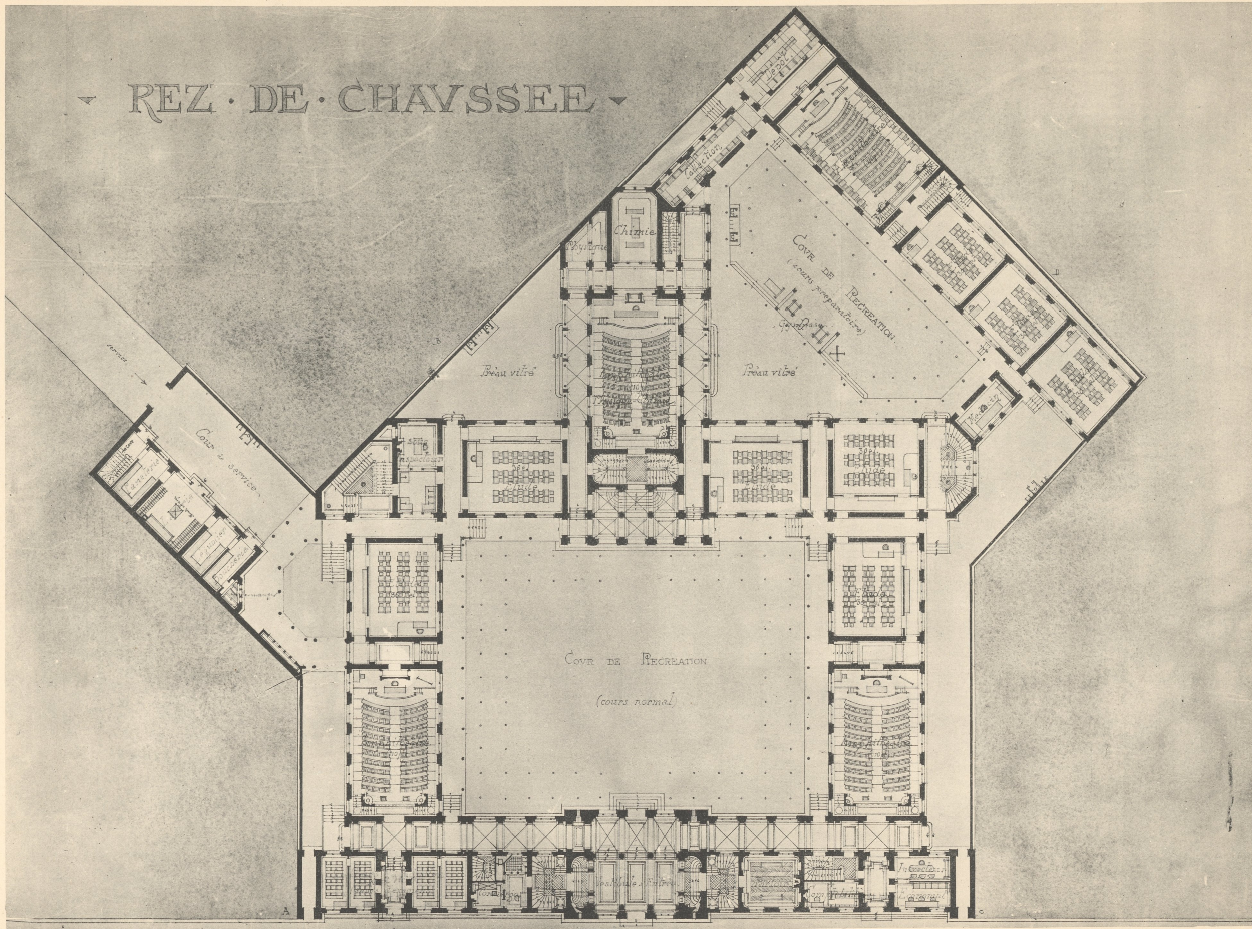
PLAN DU REZ-DE-CHAUSSEE F.-E.-L. BOUTRON & SCHOELLKOPF. - Une Ecole Supérieure de Commerce.
